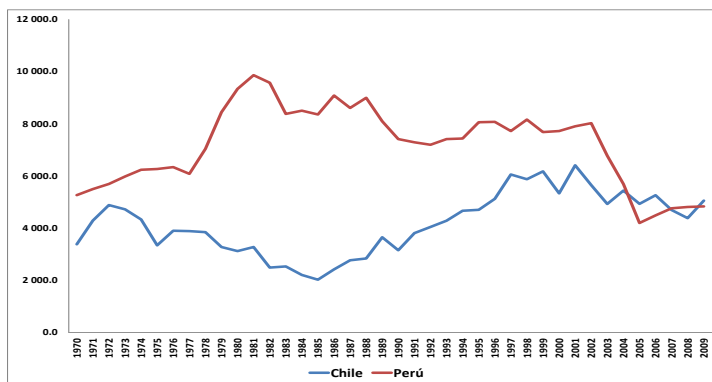
Gráfico N° 18 Producción de Kerosén y Turbo: Chile y Perú (1970-2009) (En miles de barriles equivalentes de petróleo)
